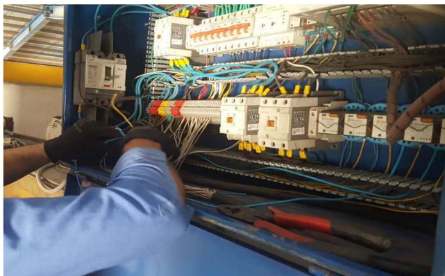
نصب حفاظت های الکتریکی در تابلو برق جرثقیل شهرک صنعتی
