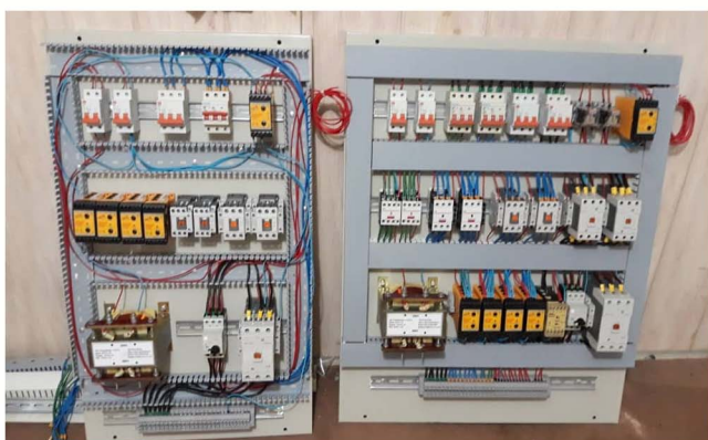
اورهال تابلو برق جرثقیل آبفا خوزستان
